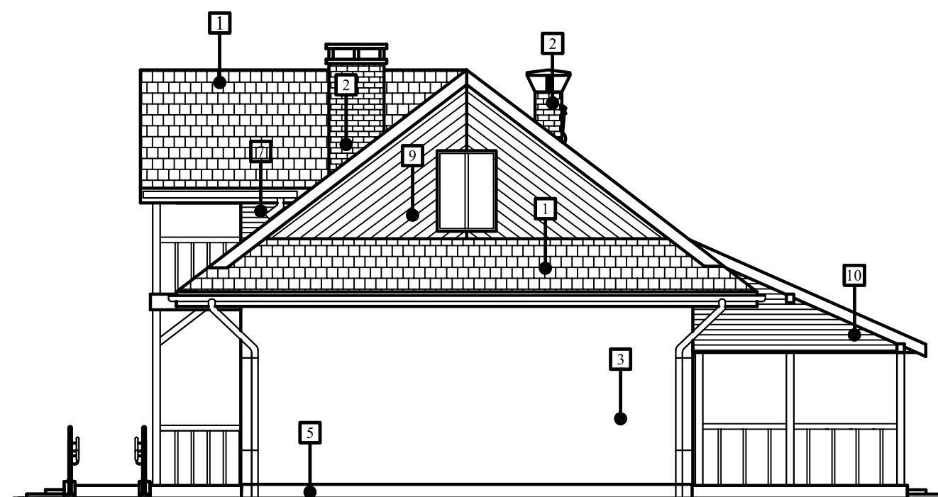
ELEWACJA WSCHODNIA
