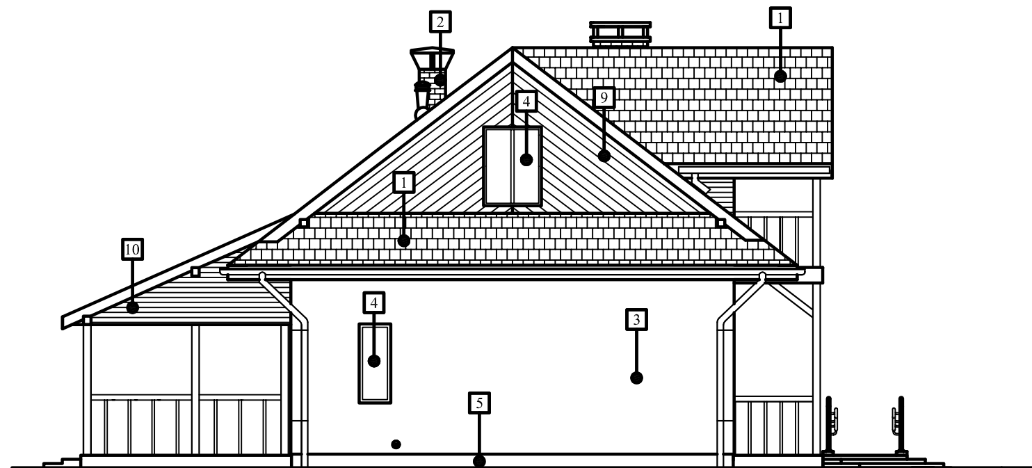
ELEWACJA ZACHODNIA
